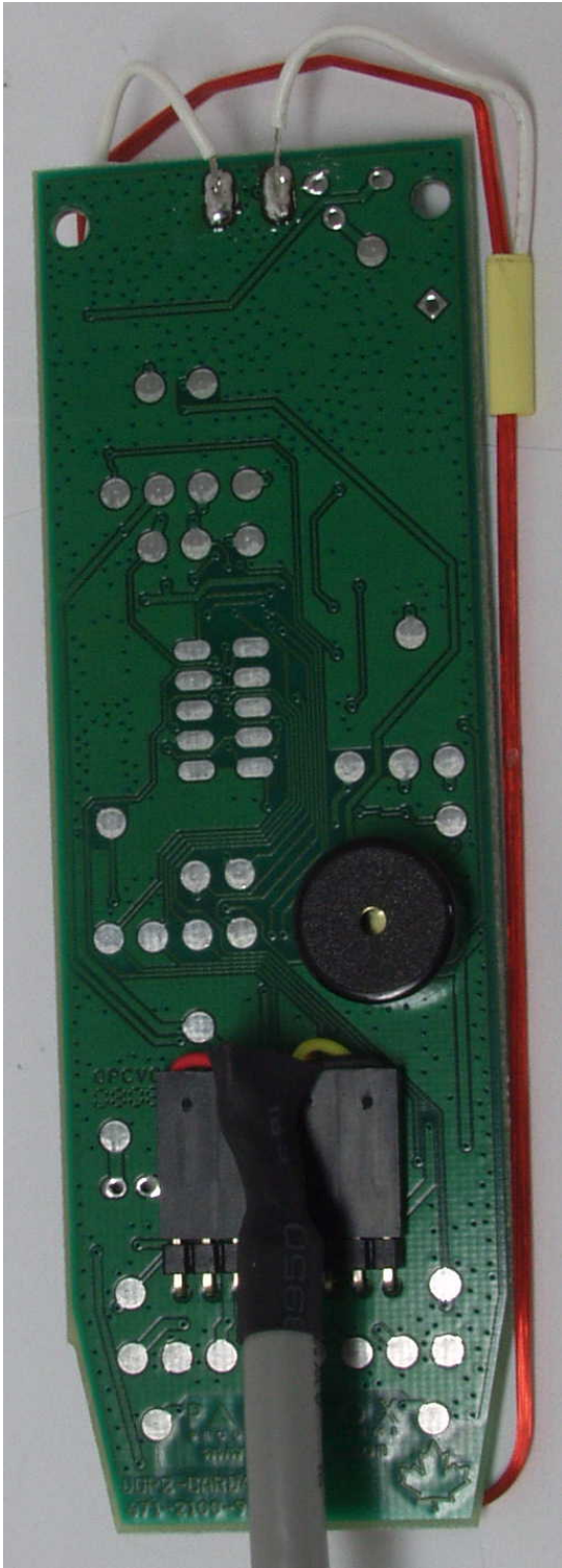
PCB-Bottom
