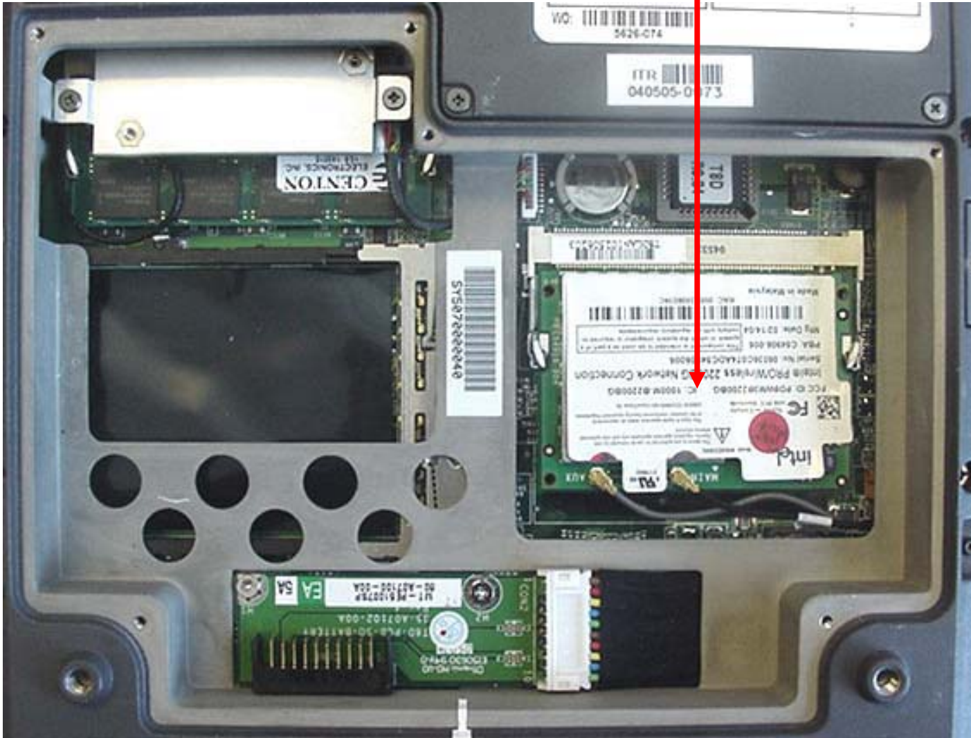
Intel Pro 2200BG 802.11b/g WLAN
