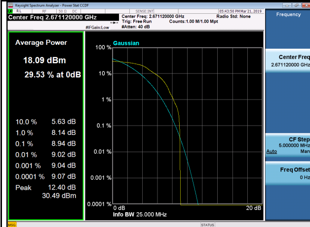
16QAM-40620
