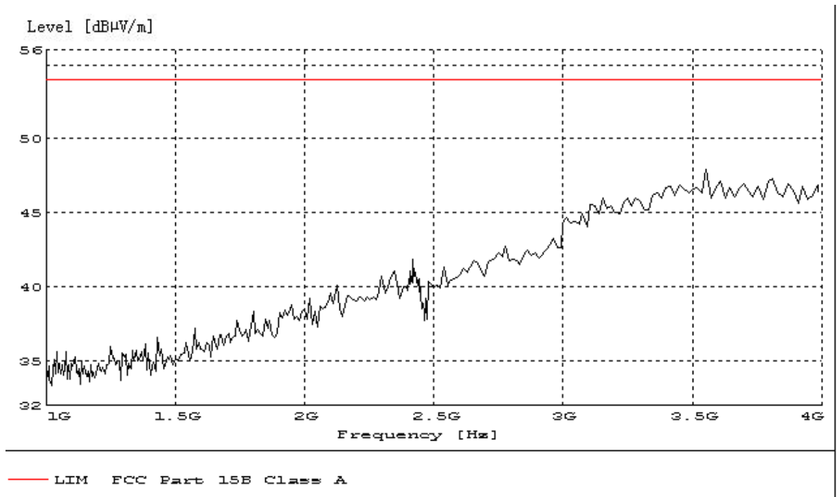
(WCDMA Band V: 1GHz-4GHz)
