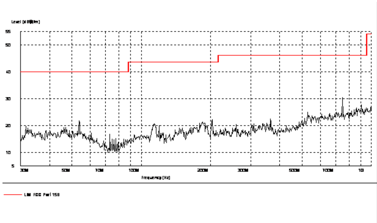
(PCS 1900MHz: 30MHz-1GHz)
