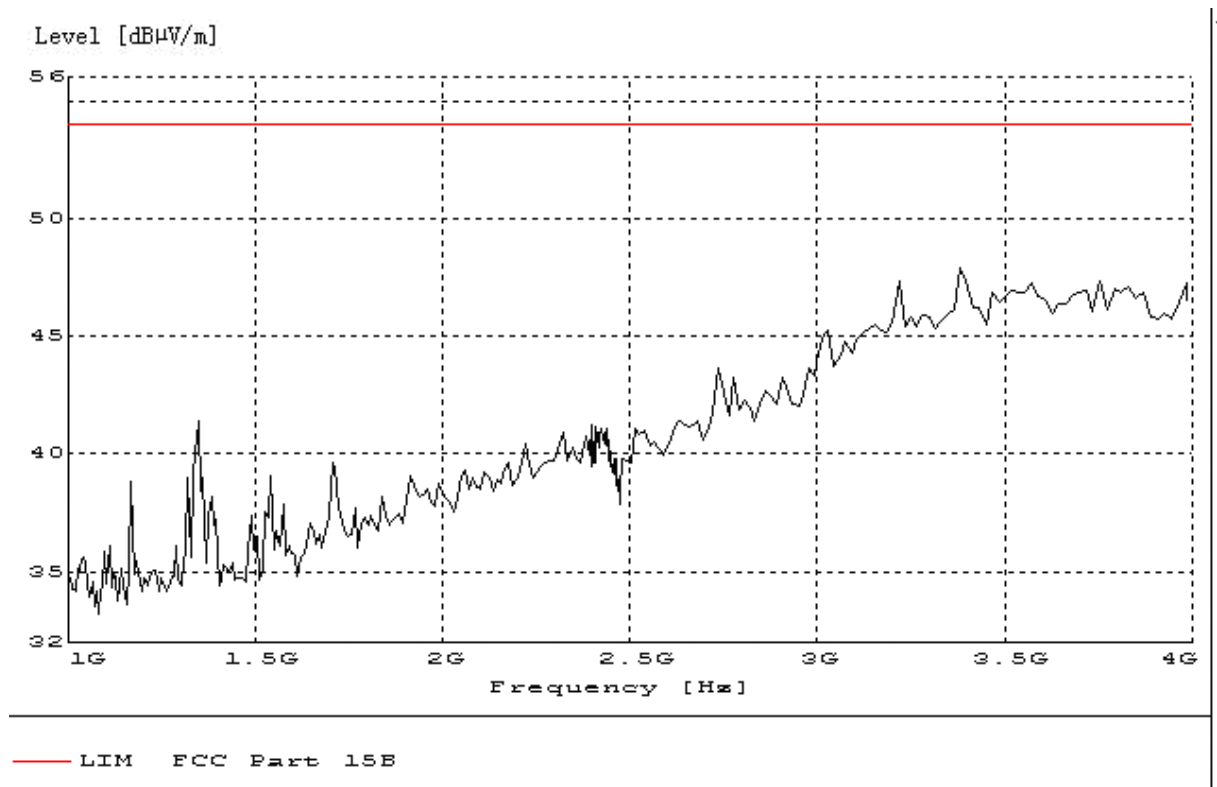
(PCS 1900MHz: 1GHz-4GHz)
