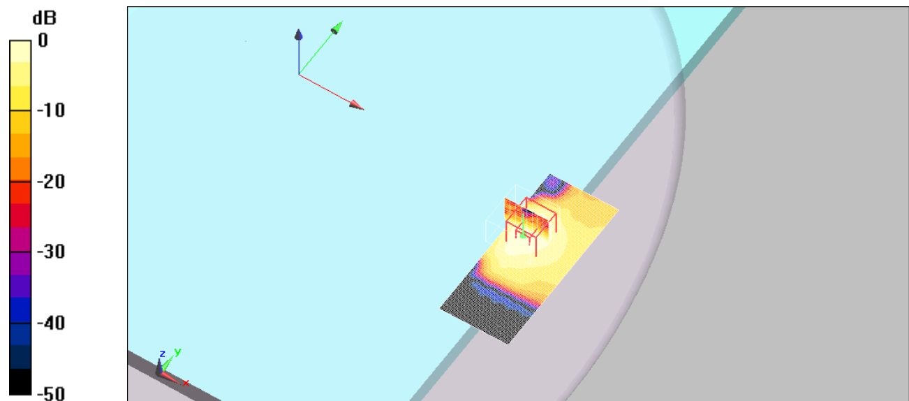
0 dB = 0.171mW/g
