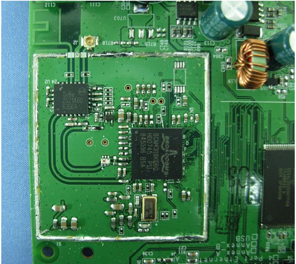
(10) EUT Photo
