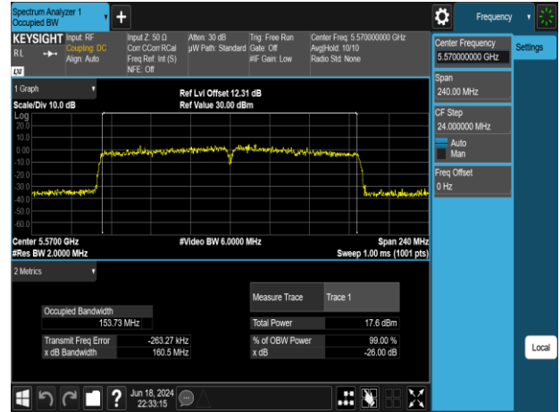
802.11ac_160MHz_Chain1_5570MHz
