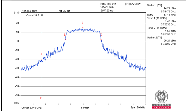
802.11a / Chain 2 : CH149
