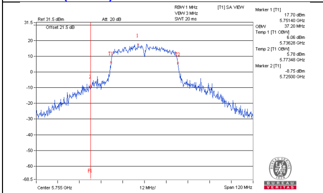
802.11ac (VHT40) / Chain 2 : CH151
