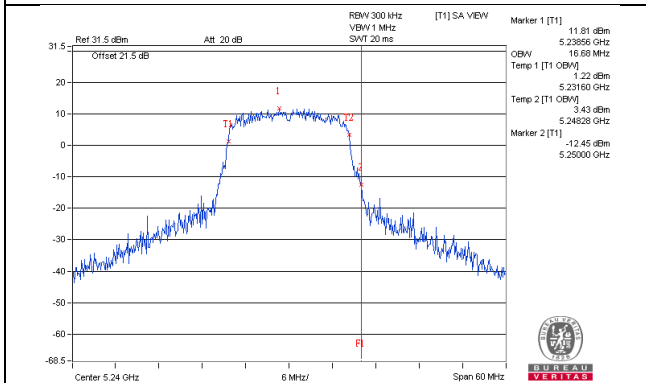
802.11ac (VHT20) / Chain 0 : CH48
