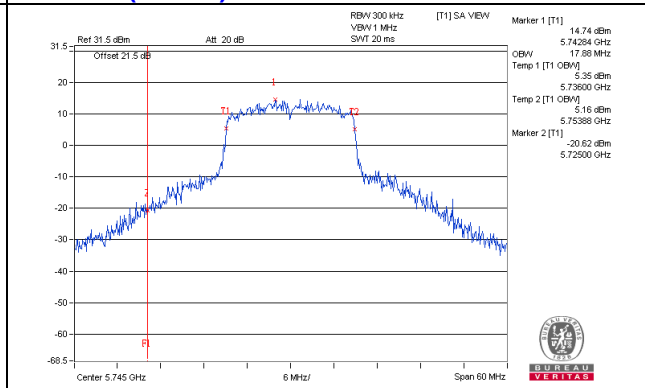
802.11ac (VHT20) / Chain 1 : CH149
