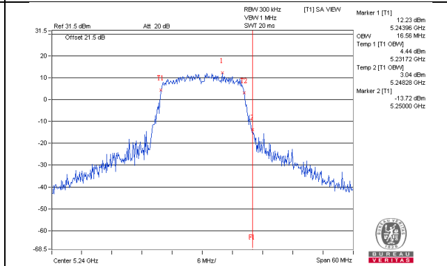
802.11a / Chain 1 : CH48
