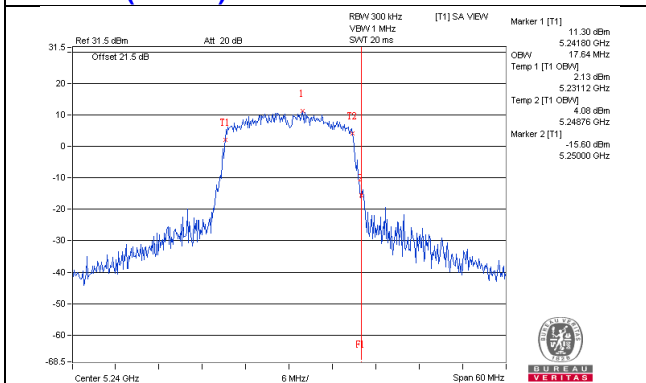
802.11ac (VHT20) / Chain 2 : CH48
