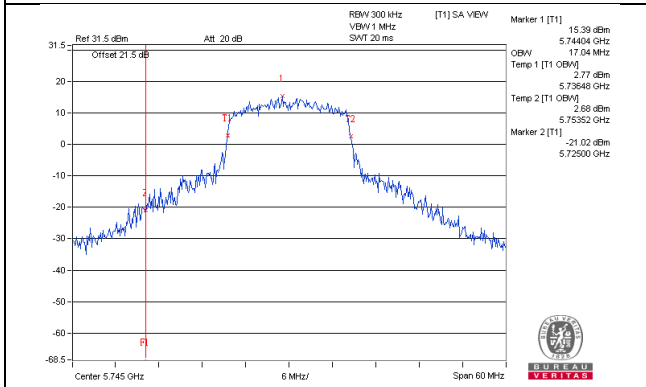
802.11ac (VHT20) / Chain 0 : CH149
