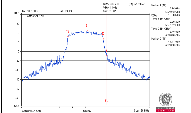
802.11a / Chain 2 : CH48
