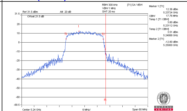
802.11ac (VHT20) / Chain 1 : CH48
