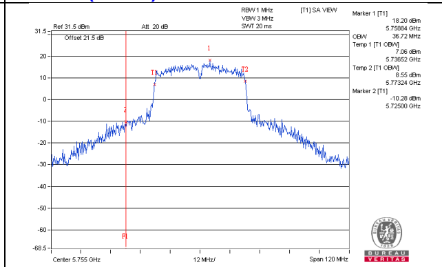
802.11ac (VHT40) / Chain 1 : CH151
