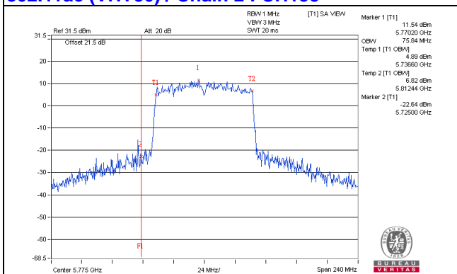
802.11ac (VHT80) / Chain 2 : CH155
