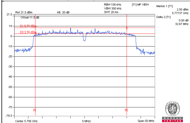
802.11ac (VHT80+80)_Chain 1 / CH155
