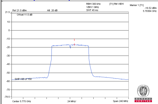
802.11ac (VHT80+80) – Chain 1: CH 155
