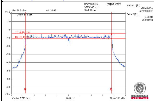
802.11ac (VHT80+80)_Chain 1 / CH155
