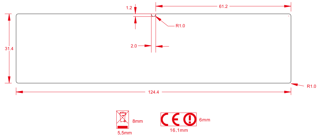
尺寸圖 outline dimension
