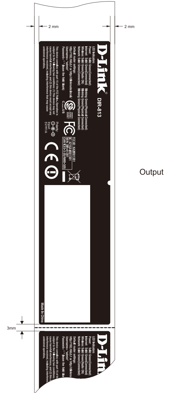
入料樣式 Incoming type
