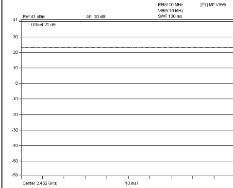
802.11n (HT20)
