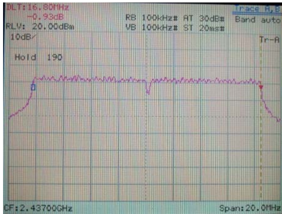
IEEE 802.11g
