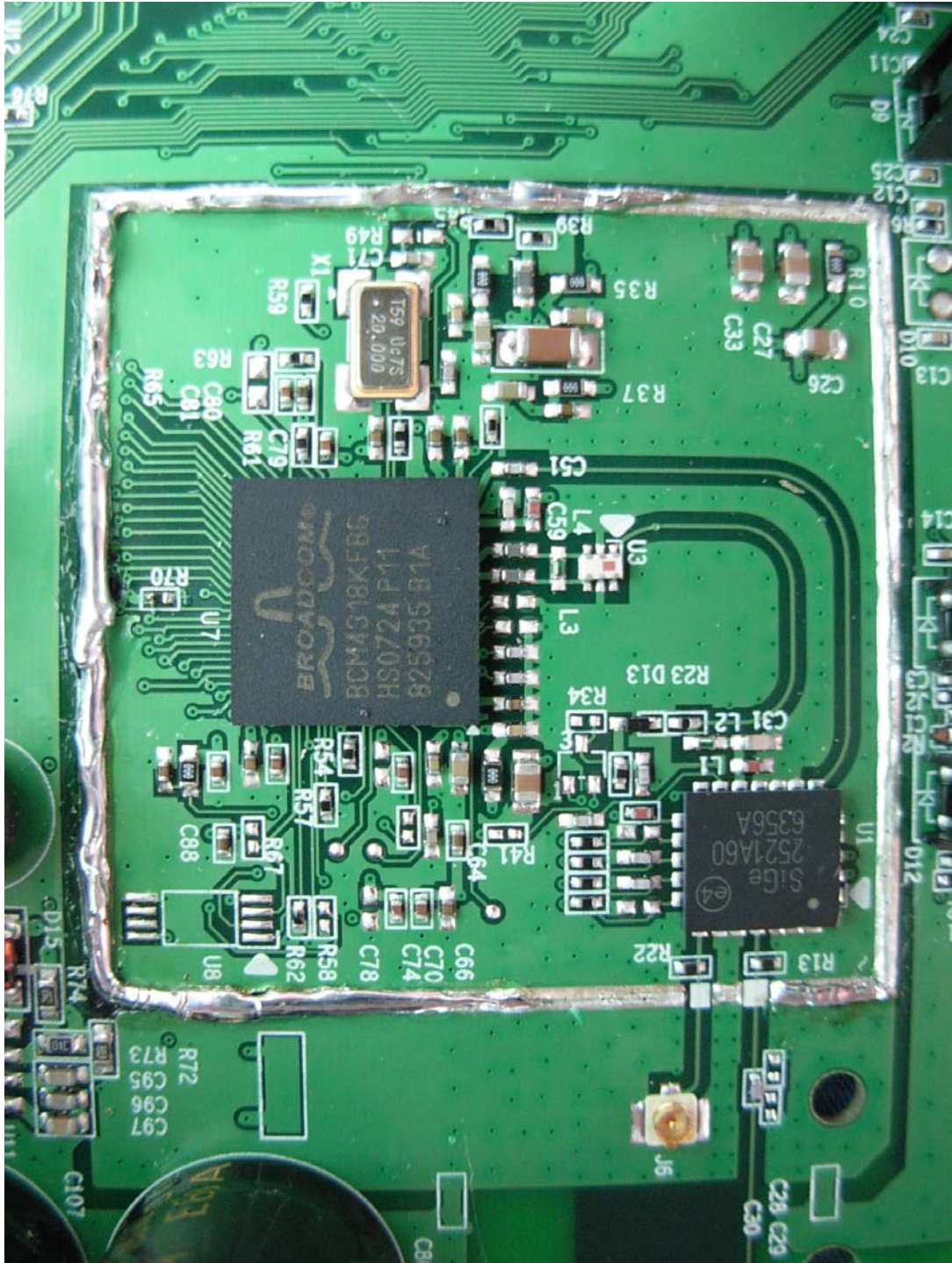
(12) EUT Photo
