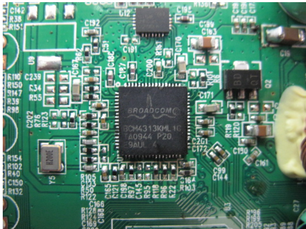
(12) EUT Photo (DSL-2730B)
