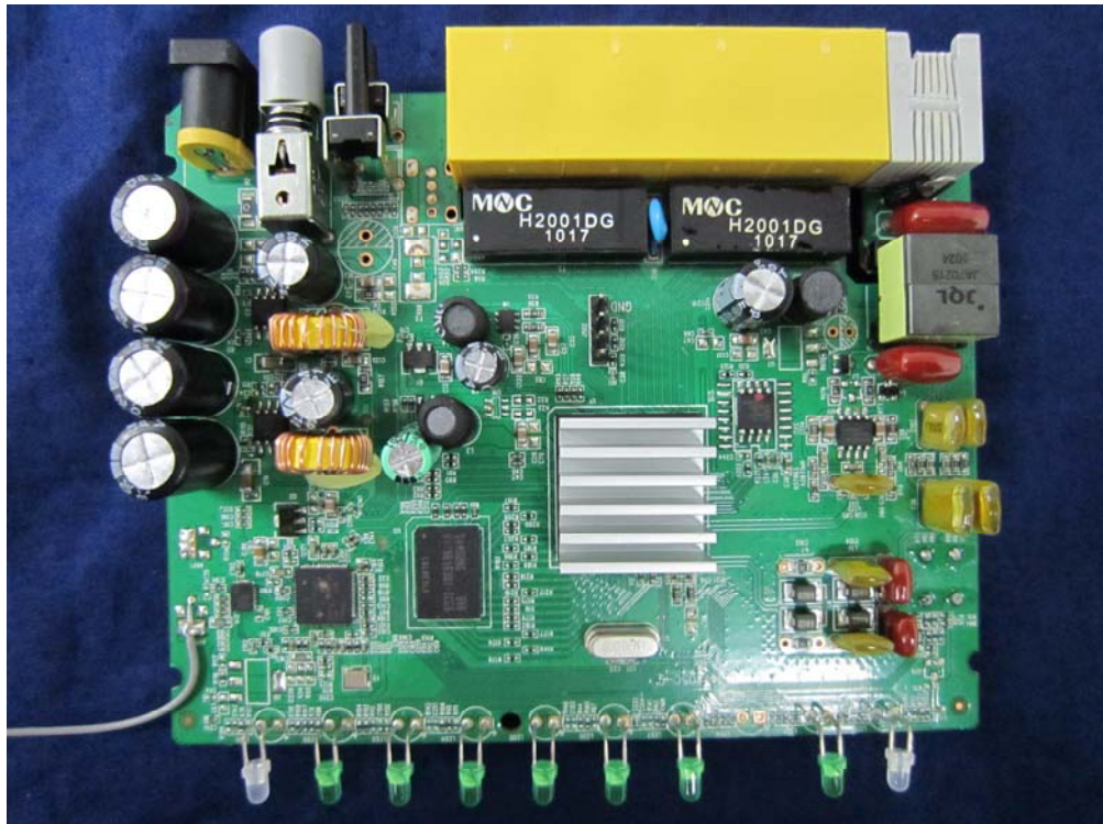
(2) EUT Photo (DSL-2640U)
