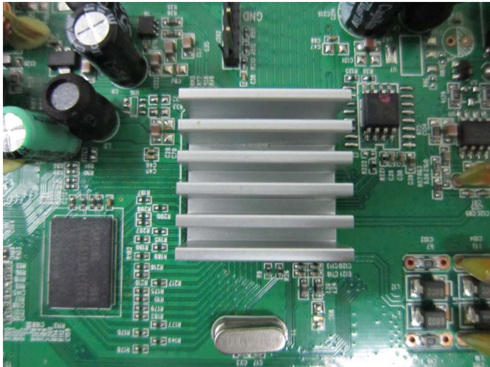
(8) EUT Photo (DSL-2730U)
