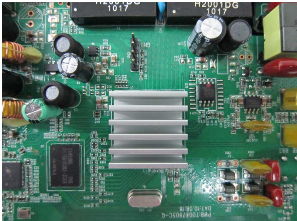
(3) EUT Photo (DSL-2640U)
