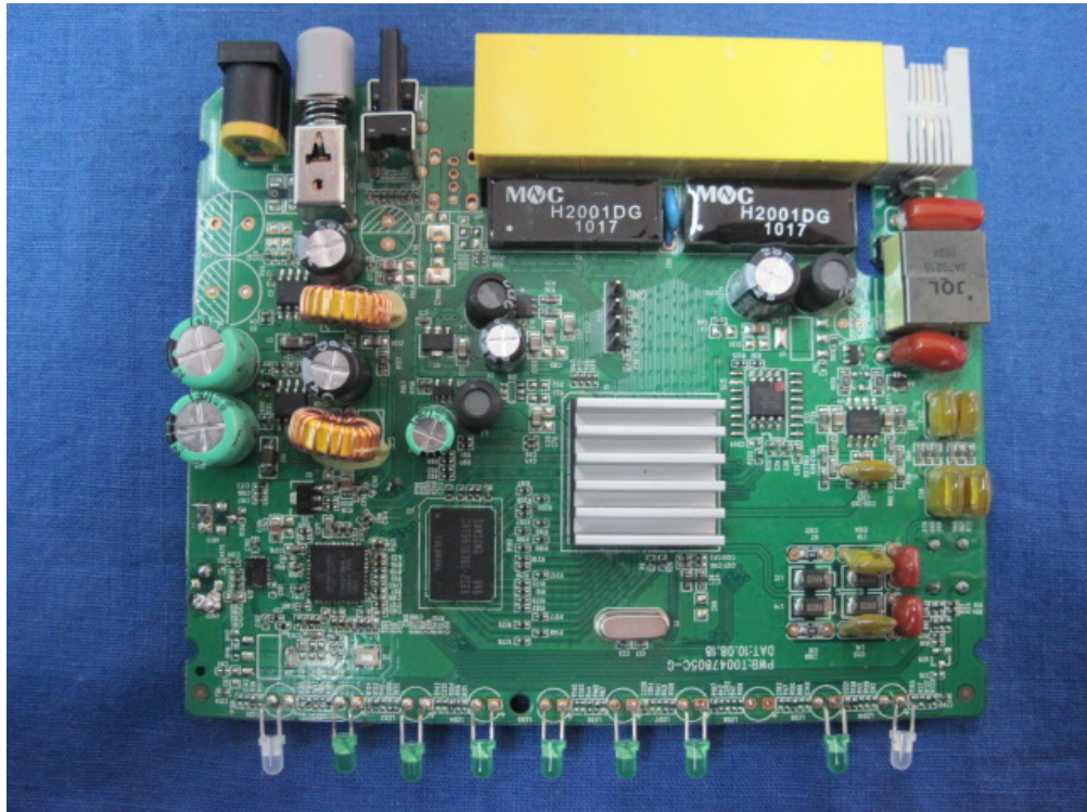
(10) EUT Photo (DSL-2730B)
