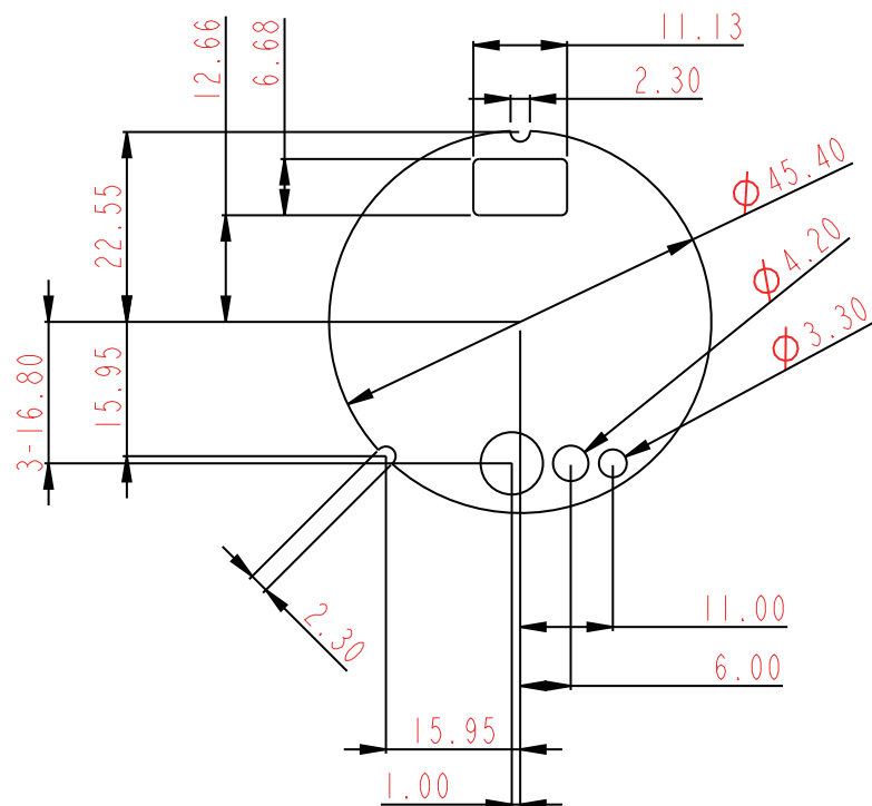
空白料尺寸圖 outline dimension for blank label
