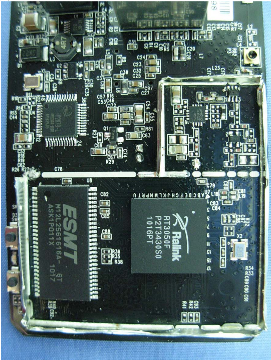
(16) EUT Photo
