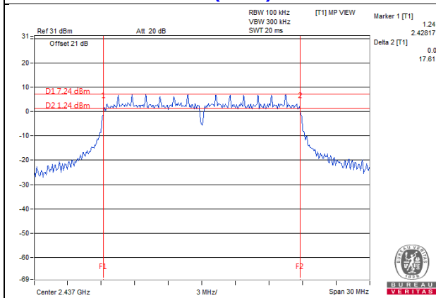
802.11n (HT20): CH6
