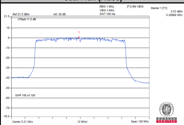
802.11ax (HE80)
