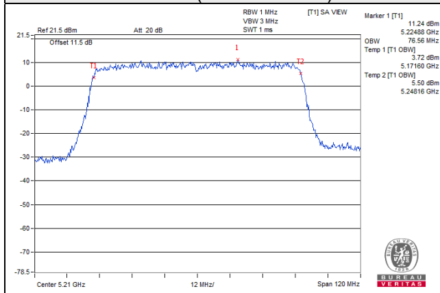
802.11ac (VHT80+VHT80)
