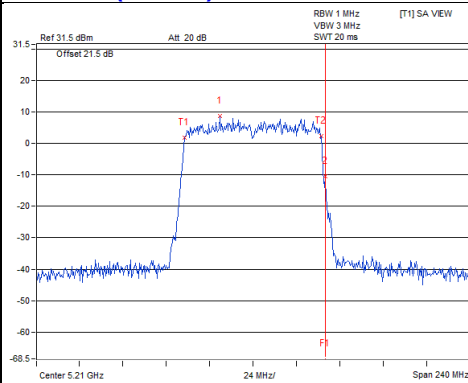
802.11ac(VHT80)_Chain2 / CH42
