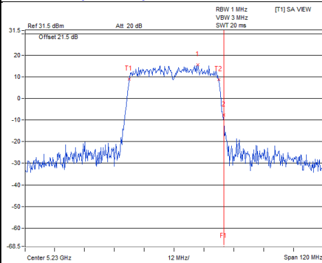
802.11ac(VHT40)_Chain2 / CH46
