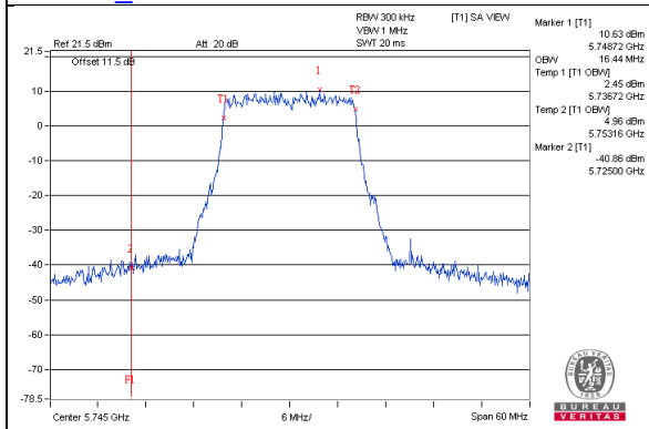
802.11a_Chain2 / CH149
