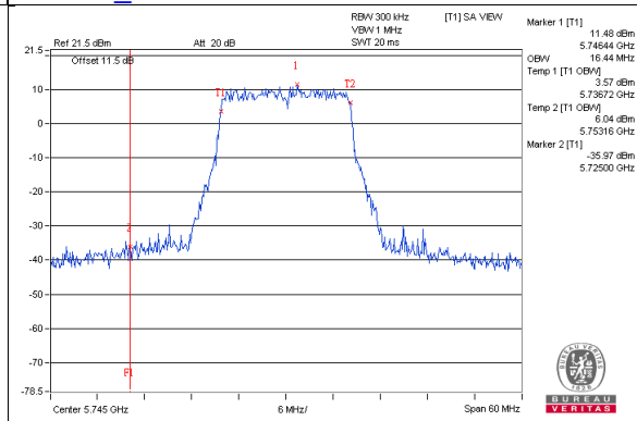
802.11a_Chain1 / CH149
