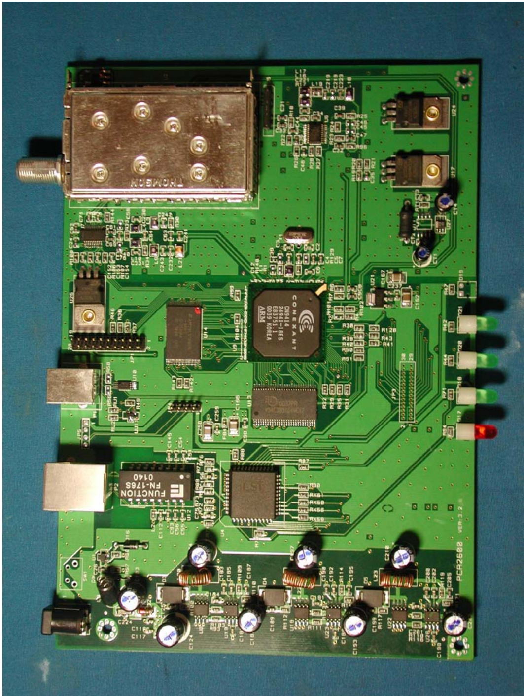
(2) EUT photo
