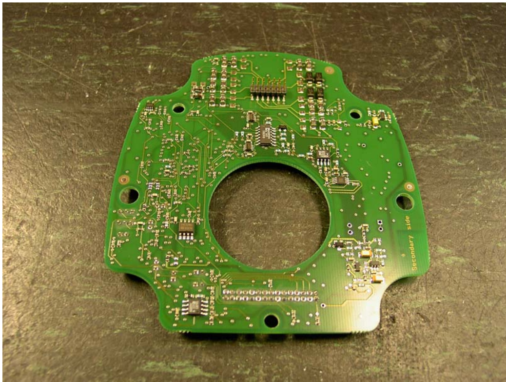
2. MB Back
