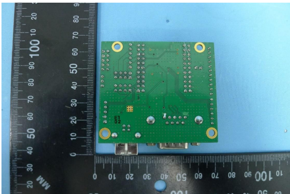
(8) UART
