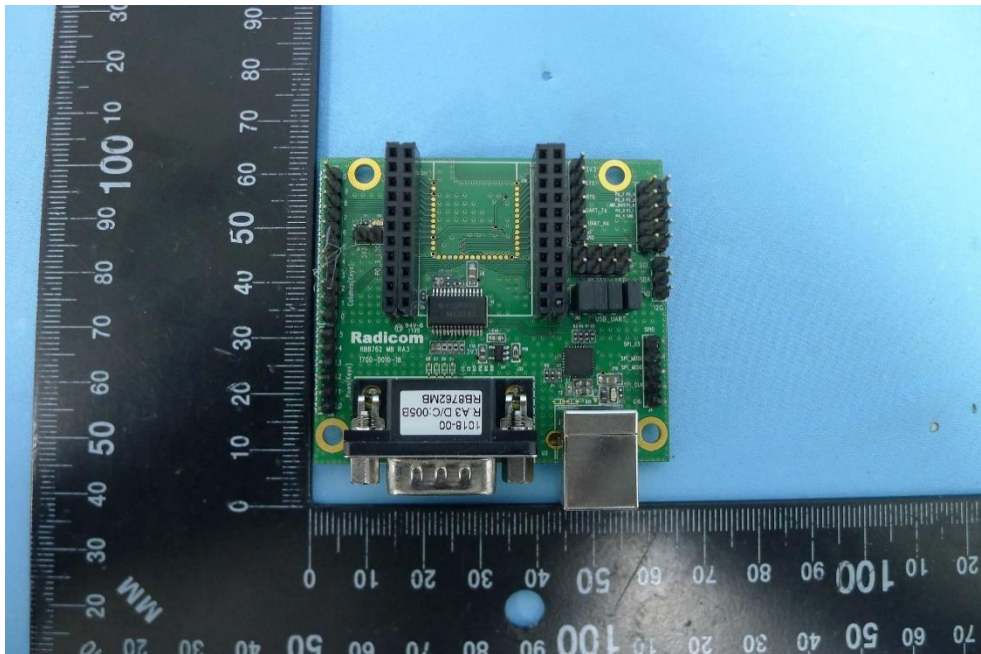
(7) UART
