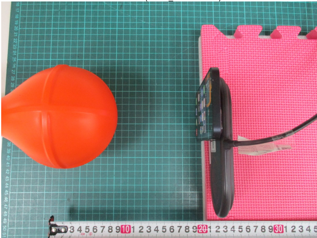
Test Mode G (Z-axis Above: 20cm)
