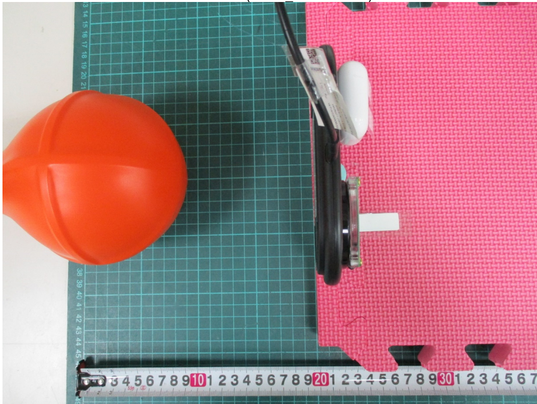
Test Mode F (Z-axis Above: 20cm)
