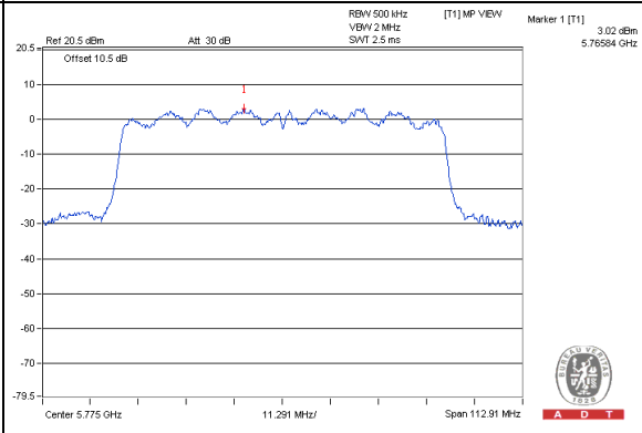
802.11ac (80MHz)
