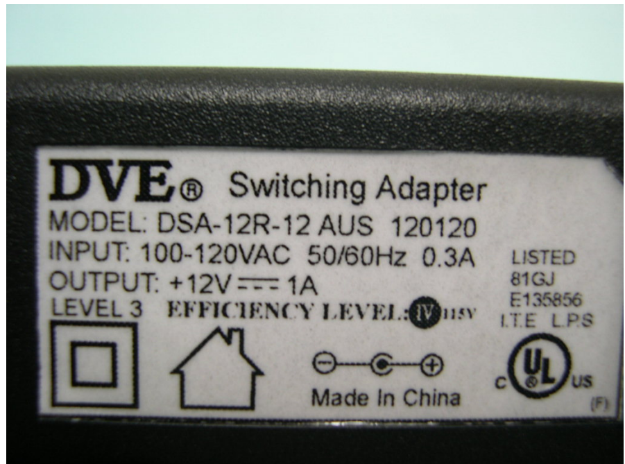
Adapter 2: DVE/DSA-12R-12 AUS 120120
