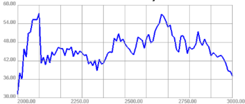
2000.00MHz - 3000.00MHz Efficiency
