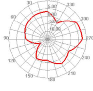
Bluetooth 39 TRP E1
