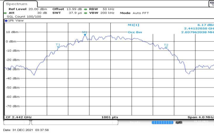
BLE_2M_Ant1_2442
