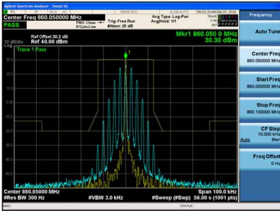
(14K0F3E _ 860.05 MHz)_Low
