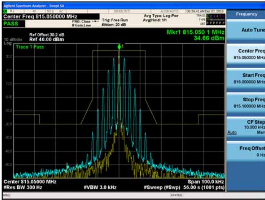
(14K0F3E _ 815.05 MHz)_High
