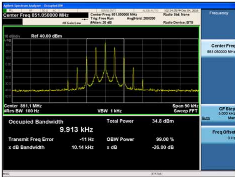
(11K0F3E _ 851.05 MHz)_High
