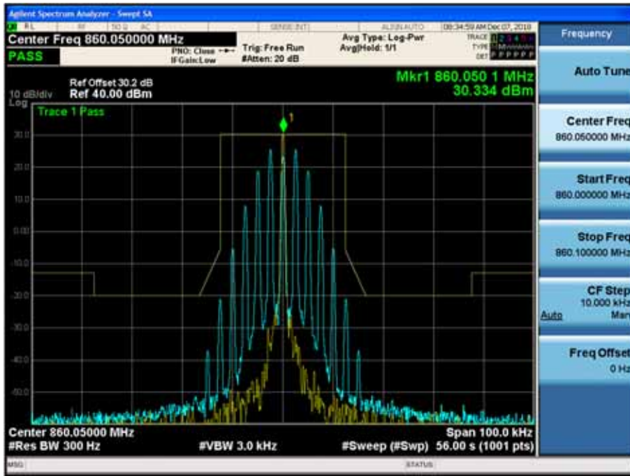
(16K0F3E _ 860.05 MHz)_Low
