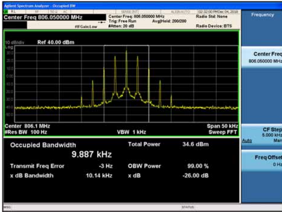
(11K0F3E _ 806.05 MHz)_High
