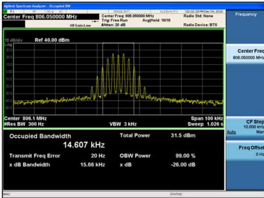
(16K0F3E _ 806.05 MHz)_Low
