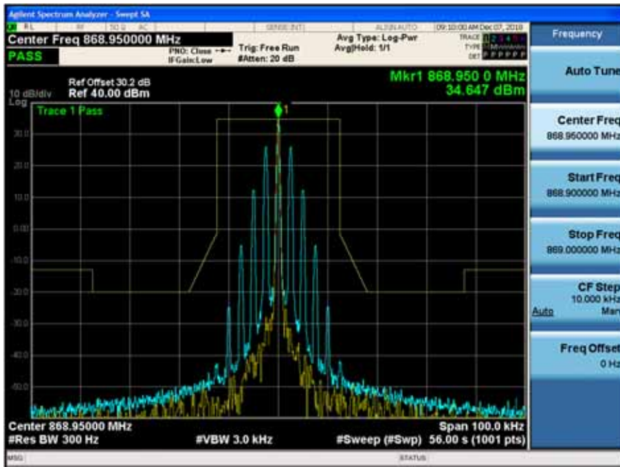
(11K0F3E _ 868.95 MHz)_High
