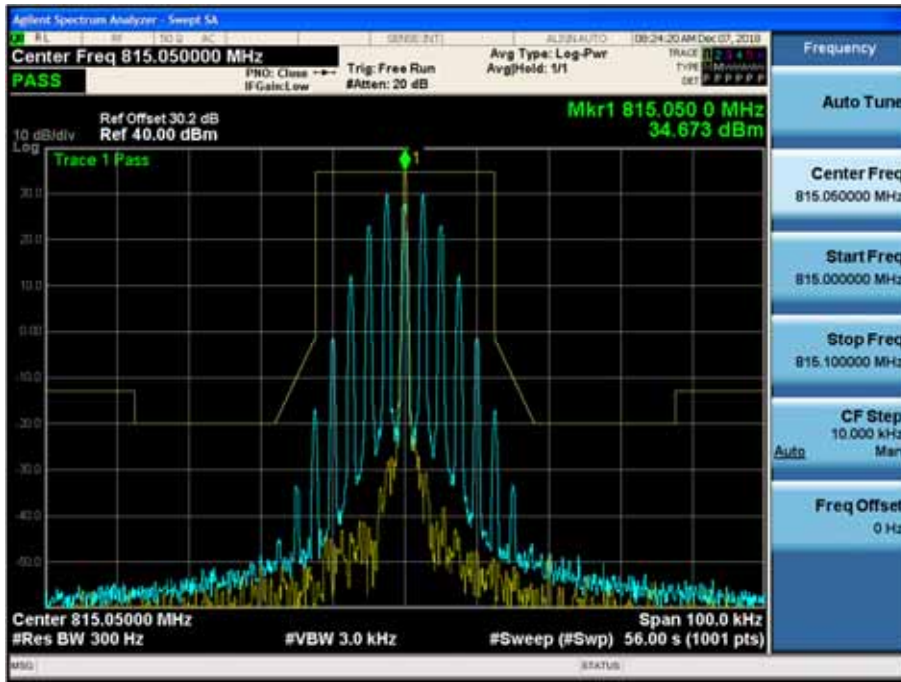
(16K0F3E _ 815.05 MHz)_High
