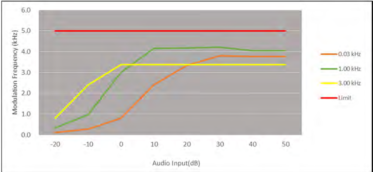
429.95 MHz
