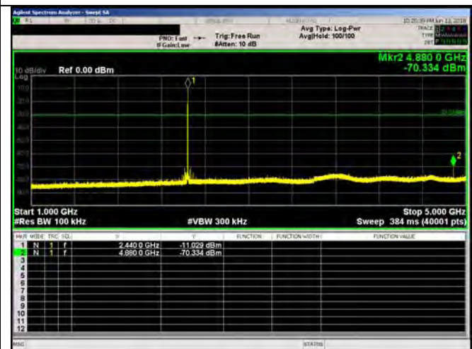
1 - 5 GHz
