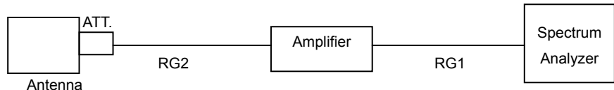
Above 1GHz(18-26.5GHz)
