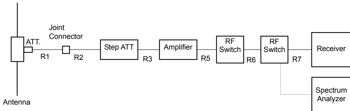
Above 1GHz(1-18GHz)
