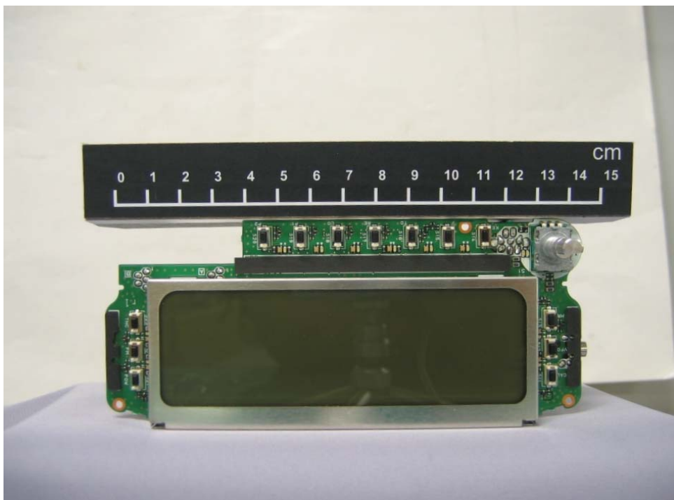
DISPLAY UNIT
