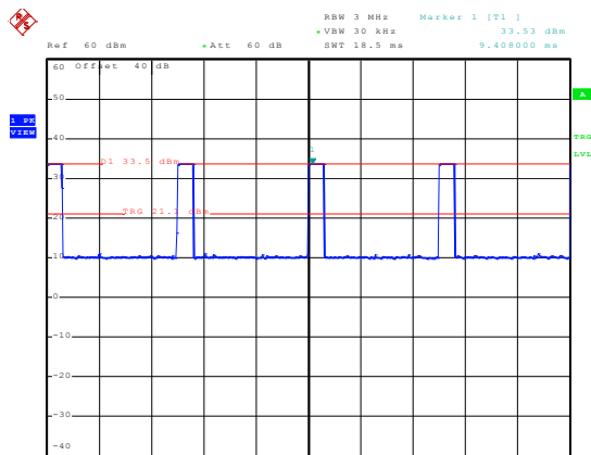
835MHz - GSM
