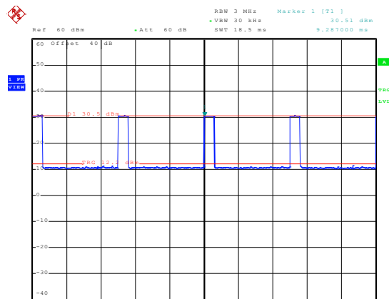
1880MHz - GSM
