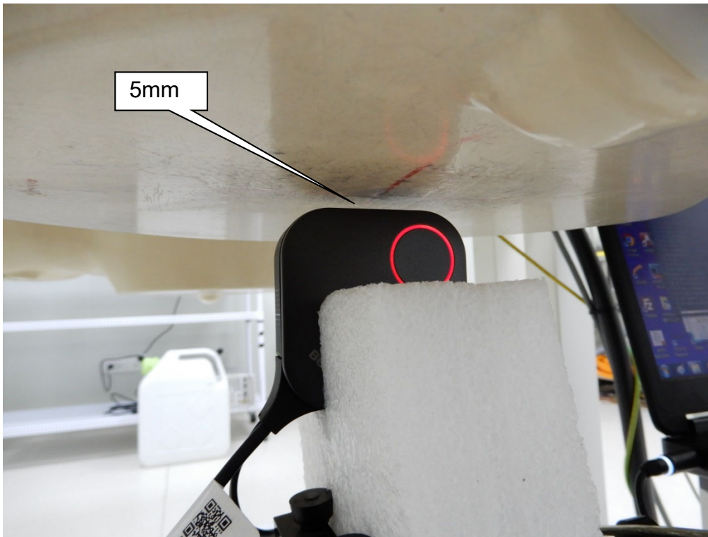
EUT Top_5mm
