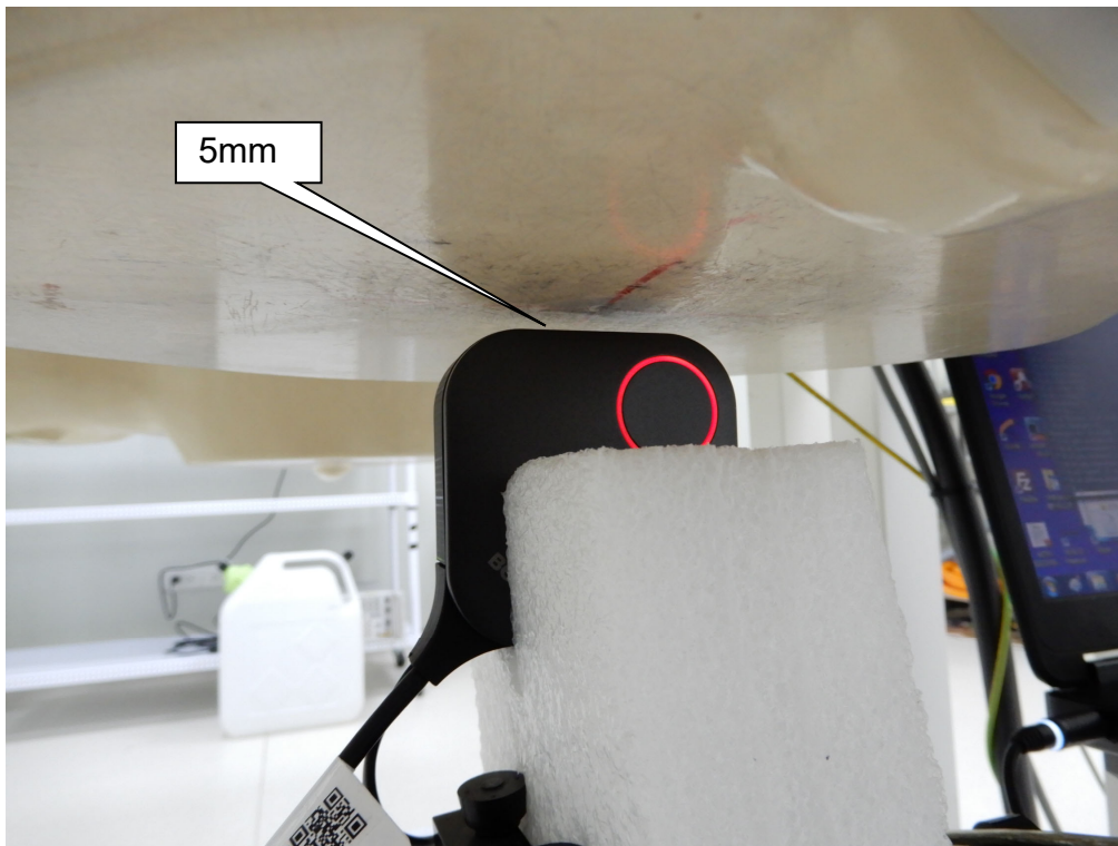
EUT Top_5mm
