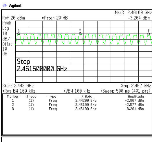
2442-2461MHz
