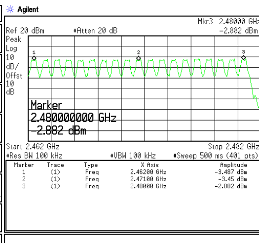
2462-2481MHz
