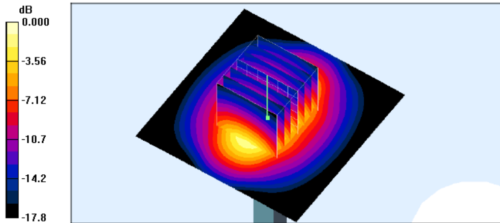
0 dB = 4.40mW/g
