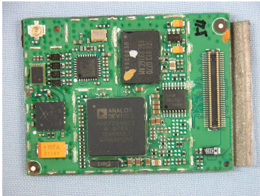
GSM/GPRS Module
