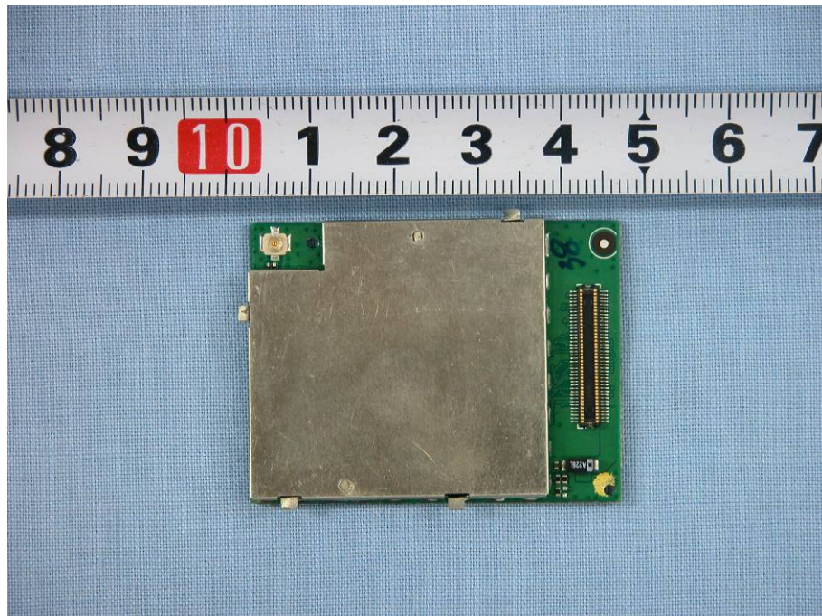
GSM/GPRS Module
