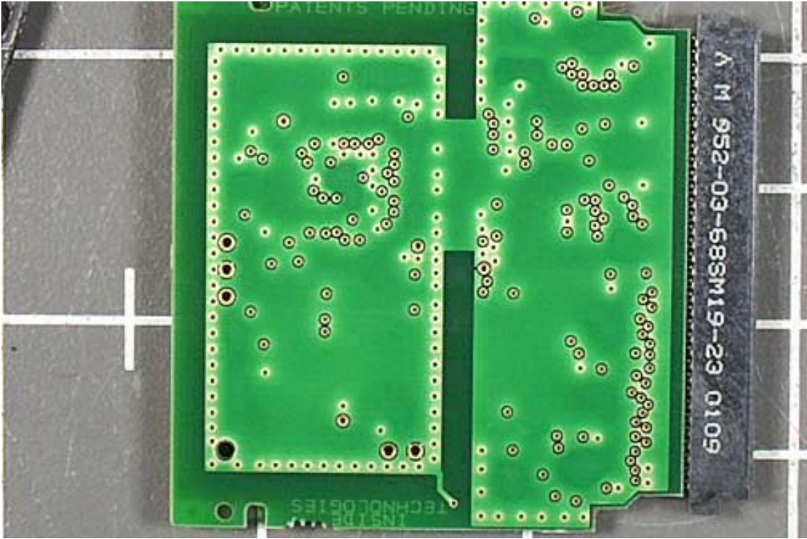
PCB 1 Bottom
