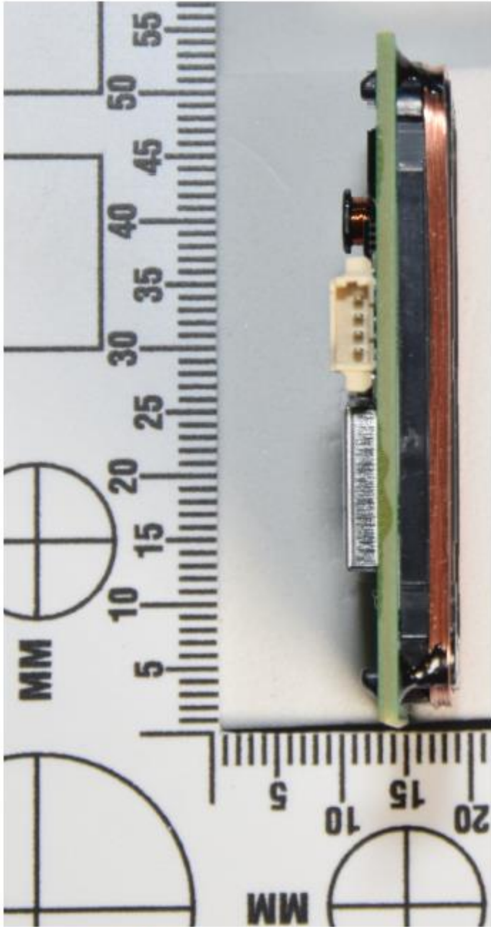
Input hopper OMNIKEY 5127CK MINI, edge 4
