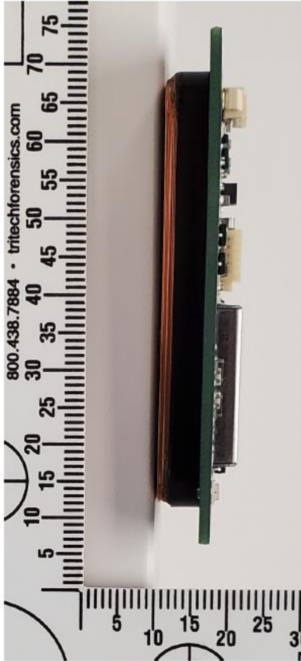
Input hopper OMNIKEY 5127CK SI, edge 3
