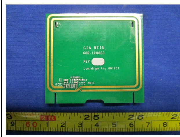
PCBA 2(ANTENNA) Bottom View3
