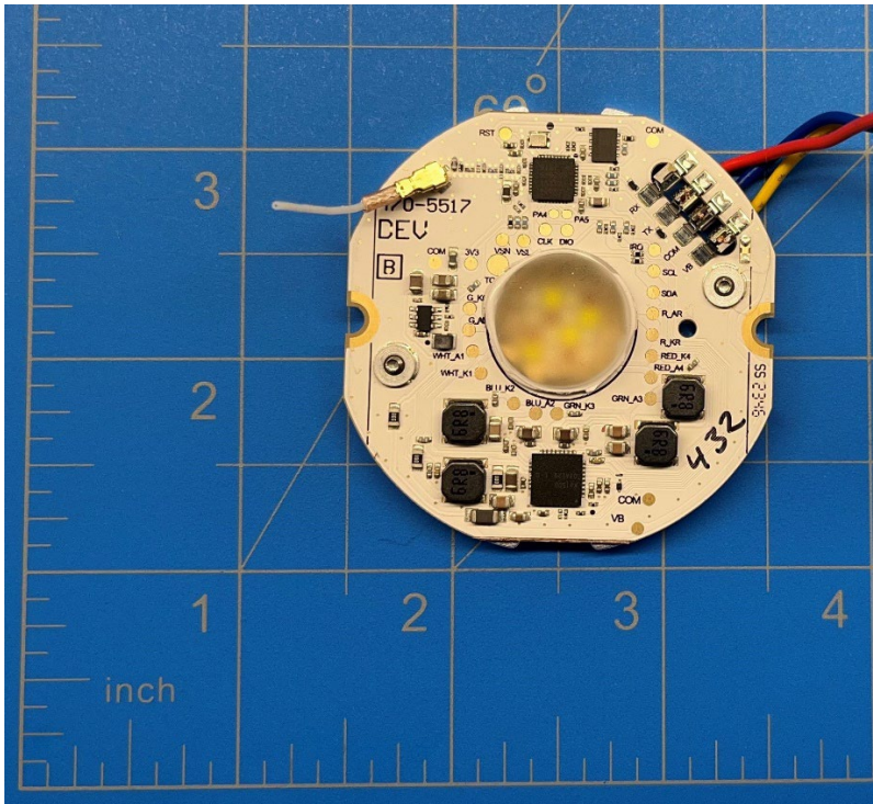
Bottom Side
