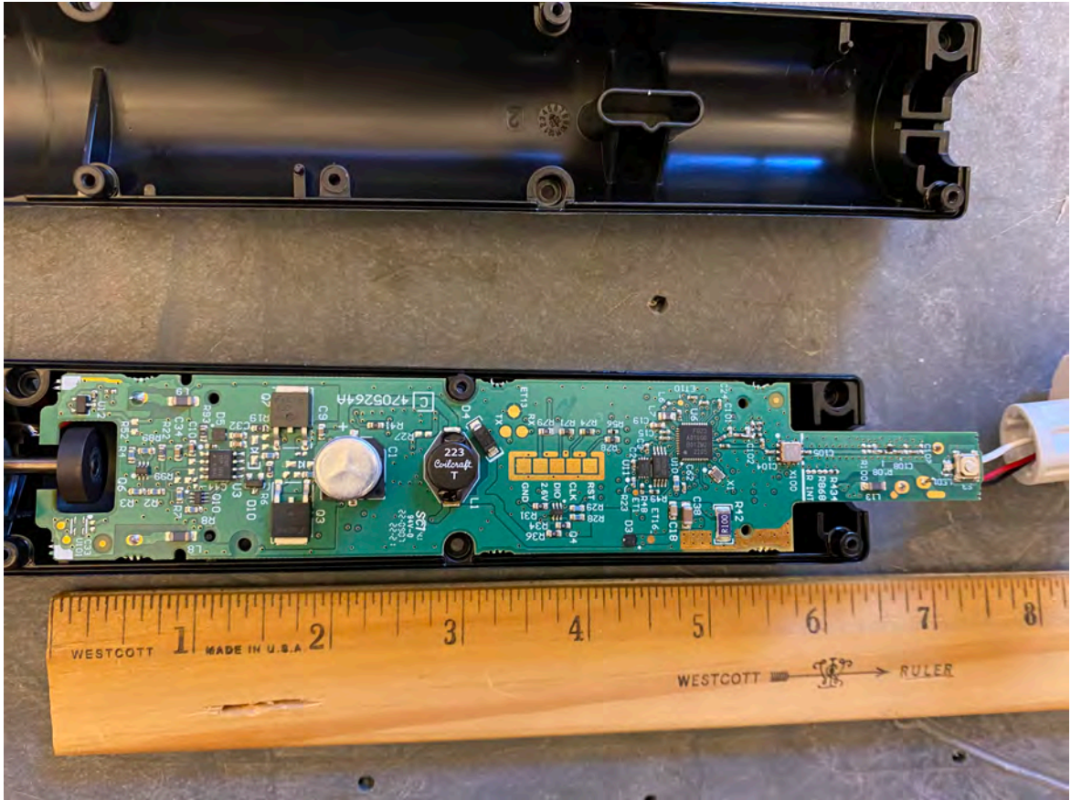
Top PCB
