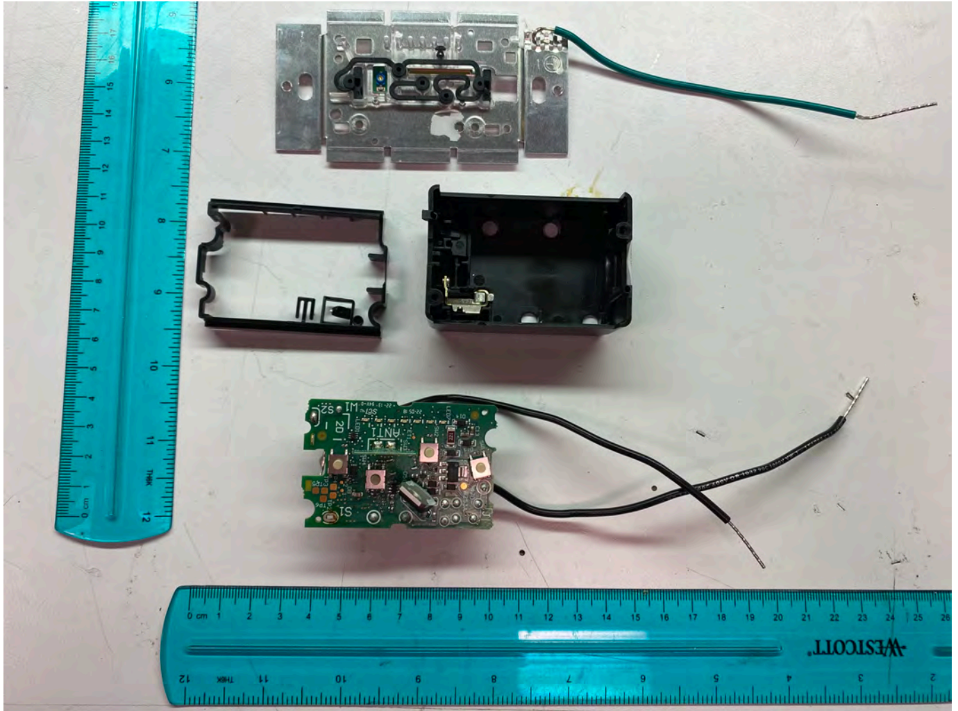
Top PCB
