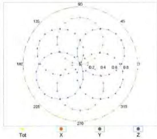
f=1800 MHz,R22
