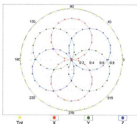
f=1800 MHz,R22
